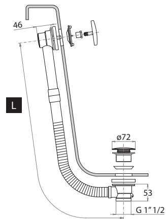
Colonna di scarico per vasca in ottone/rame Bath "Skip-up" waste & overflow in brass/ copper
