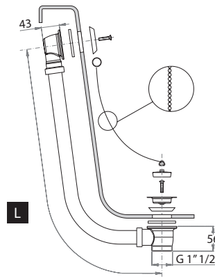
Colonna di scarico per vasca in ABS con tappo a catenella per vasche a vista ABS bath waste & overflow with plug and chain for exposed bathtubs
