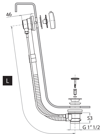
Colonna di scarico per vasca in ottone/rame Bath pop-up waste & overflow in brass/copper
