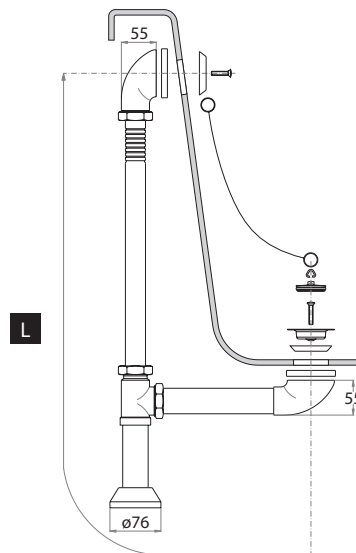
Colonna di scarico per vasca in ottone con tappo a catenella per vasche a vista, modello "America" Brass bath waste & overflow with plug and chain for exposed bathtubs, "America" model
