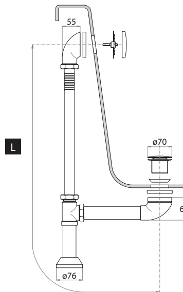
Colonna di scarico per vasca in ottone con sistema di comando "Skip-up" per vasche a vista, modello "America" Bath pop-up waste & overflow in brass with "Skip-up" plug system for exposed bathtubs, "America" model
