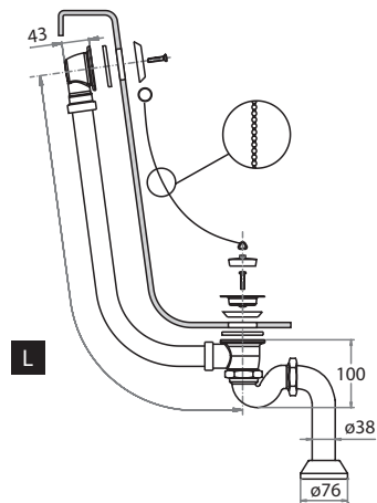
Colonna di scarico per vasca in ABS con tappo a catenella per vasche a vista ABS bath waste & overflow with plug and chain for exposed bathtubs
