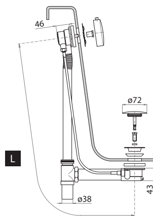
Colonna di scarico per vasca modello "America" • Trasmissione con movimento "Direct" Bath pop-up waste & overflow "America" model • "Direct" drive system
